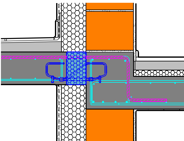
Balkon v višji višini
