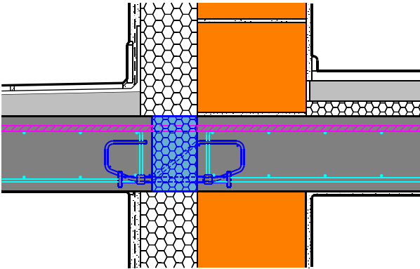
Balkon v isti višini
