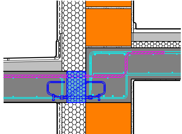
Konzolna stenska plošča
